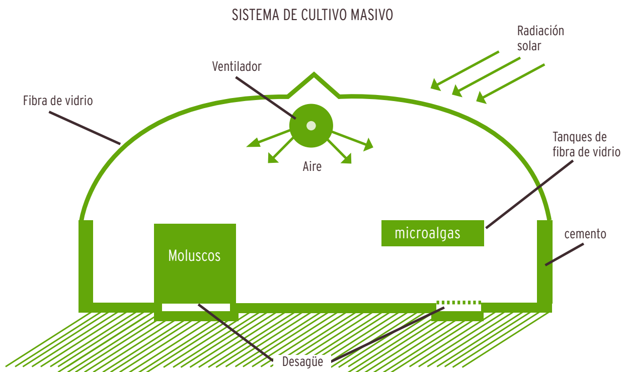
► ESQUEMA DEL INVERNADERO DE WACHAPREAGUE (USA). CULTIVO MASIVO CON TEMPERATURA CONTROLADA EN INVERNADERO CON VENTILADOR
